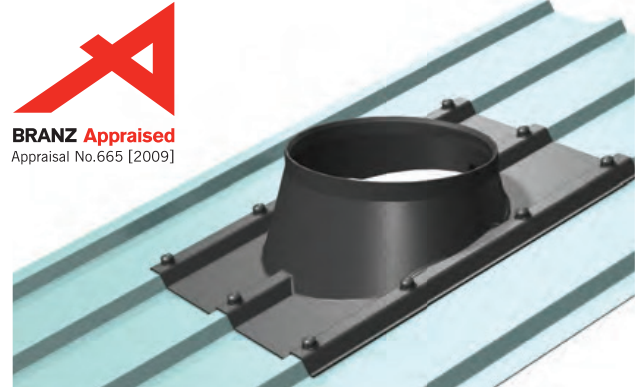
Trimdek
